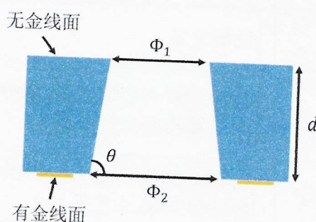
图3 侧壁陡直度的定义
